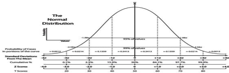
شکل ۲: منحنی نرمال
